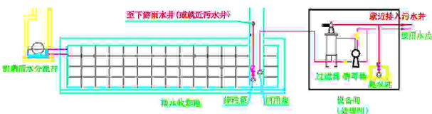
工艺流程图
