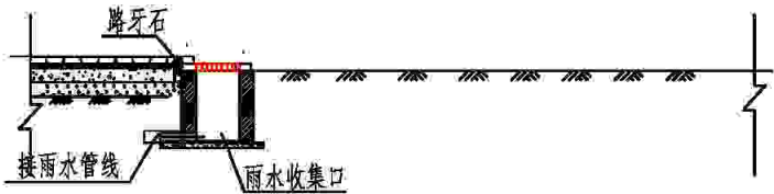
A-A剖面图 1:40
