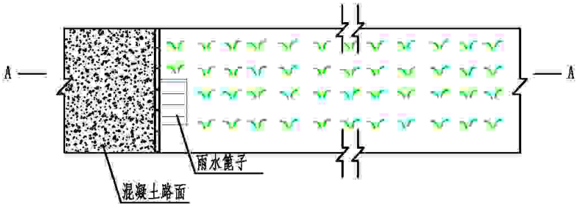
下沉式绿地平面设计图 1:40
