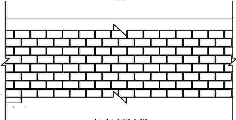
生态透水砖铺装平面图 1:20
