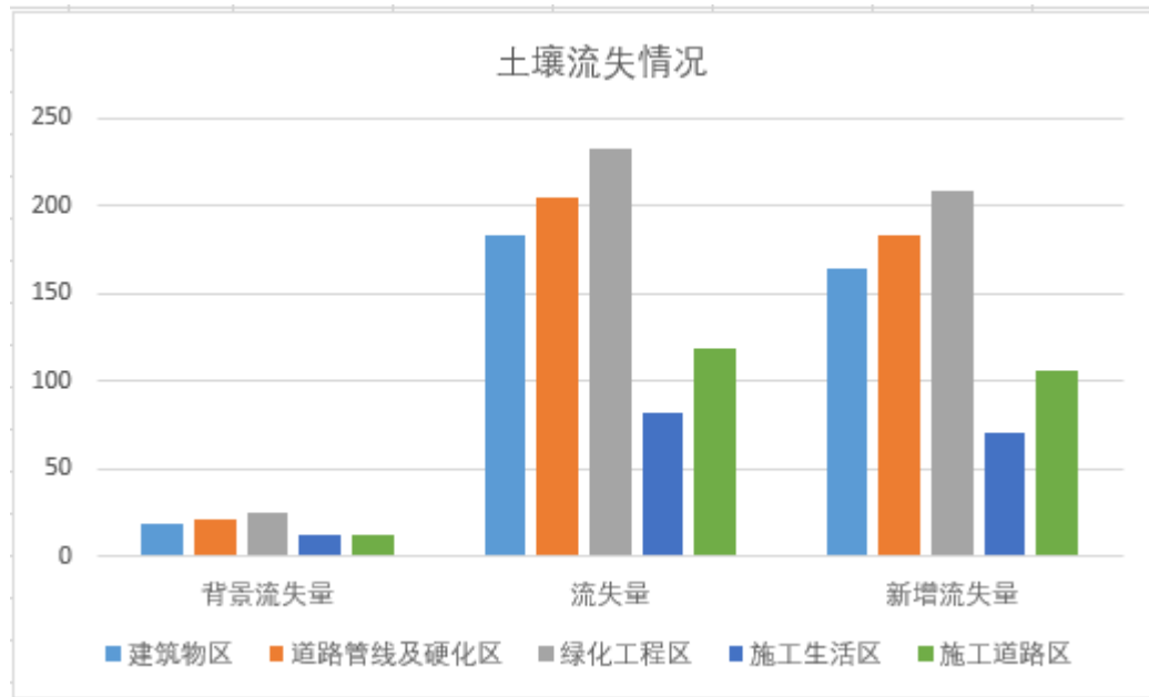
图4-1 土壤流失量的分布图
