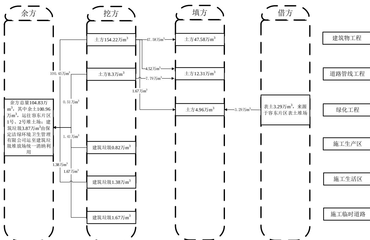
图2-16 土石方流向图
