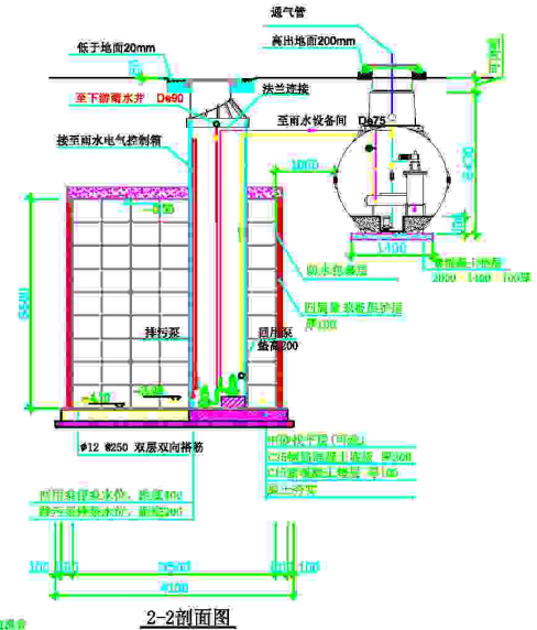
2-2剖面图
