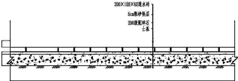
生态透水砖铺装断面图 1:20
